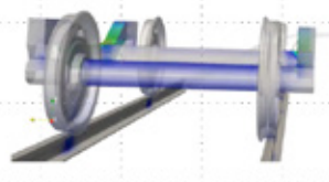
車輪・レール間接触 Rail-wheel contact
