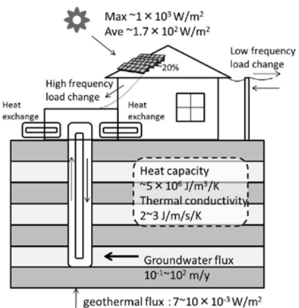
地中熱ヒートポンプシステムによる負荷平準化の可能性 Possibility of electric load levelling by geothermal heat pump system
