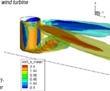
スパー型浮体式洋上風車 Spar-type floating offshore wind turbine
