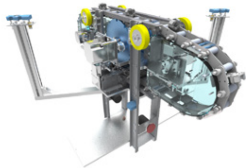
HanGrawler: 無限軌道機構を用いた天井移動ロボット HanGrawler: Large-payload and high-speed ceiling mobile robot using crawler
