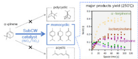
固体酸触媒を利用した高温高压水中の有機合成 Organic synthesis in hot compressed water using solid acid catalyst
