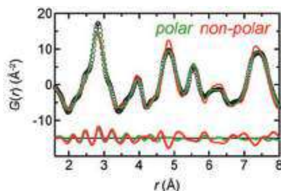
中性子を用いた2体相関分布関数解析 (左) から導き出した高誘電体 LaTiO 2 N の極性 (polar) ナノ構造 (右)。矢印は非極性 (non-polar) 構造からの変位を示している。
