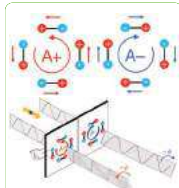
図3:電気双極子の渦状配列(フェロアキシャル秩序)とそこで実現する電気旋光性の概念図。
