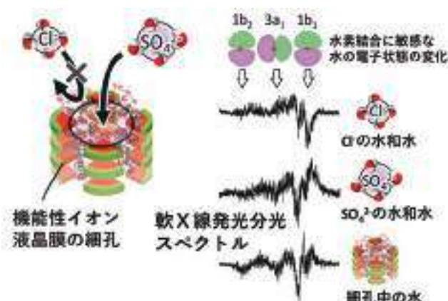
図:機能性イオン液晶膜は、極めて均一かつナノメートル程度のサイズを持つており、透過させるイオンを選ぶ機能がある。軟X線発光分光を用いて機能性イオン液晶膜が取り込む水を調べた結果、イオンを取り巻く水の水素結合構造が穴の中でも安定に存在することが、イオンを選択的に通す条件の一つとなることを見出した。
