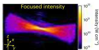
図1: X線レーザー光を7 nmのサイズに集光することで世界最高強度( 10^{22} W/cm 2 )のX線パルスの生成に成功した。
