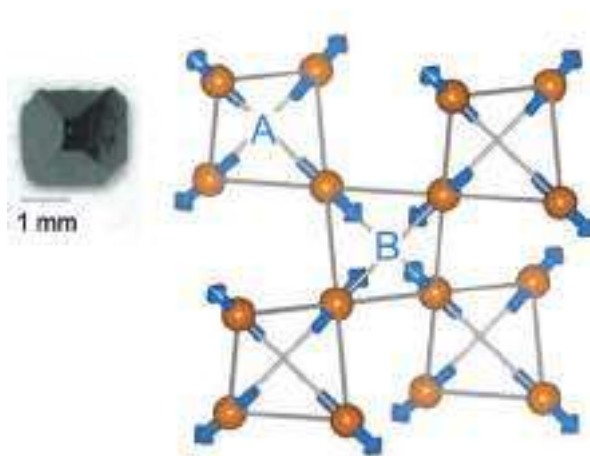
Cd 2 Os 2 O 7 単結晶において-46℃以下で出現するall-in-all-outと呼ばれる非常に対称性の高い美しいスピンの配列。放射光共鳴X線磁気散乱で明らかにされた。
