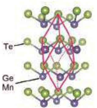
強磁性ラシュバ半導体 (Ge,Mn)Te の結晶構造
