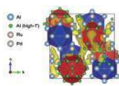
アルミニウム原子の拡散経路 (黄) と、高次元空間の揺らぎで出現する仮想アルミニウム原子 (緑)
