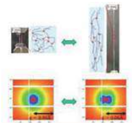
高強度ゲルの延伸に伴う小角散乱パターンの変化
