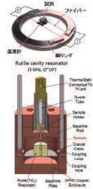
図3: 長時間緩和法による精密比熱測定(上図)とルチル空洞共振器によるマイクロ波測定(下図)
