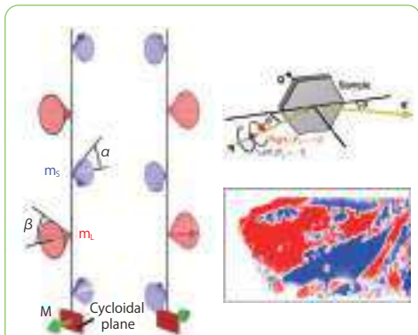
図1:室温マルチフェロイック物質のらせん磁気構造と円偏光共鳴X線回折で観測されたそのドメイン構造。
