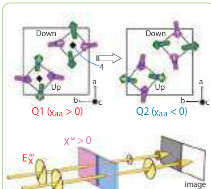
図2:電気磁気効果を示す銅化合物の磁気四極子秩序とそこで実現する電気磁気光学効果の概念図。
