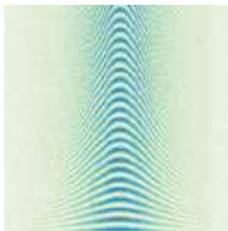
単一電子スピン量子状態の高忠実度操作
