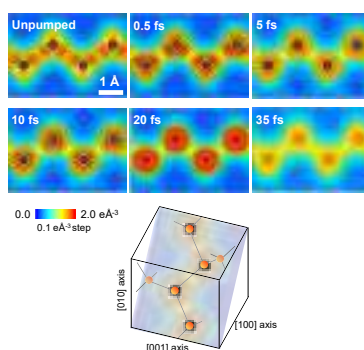
図2: X線を照射後のダイヤモンドの電子密度分布の変化。結晶構造を保ったまま、化学結合が消失したエキゾチックな物質の状態が実現されている。
