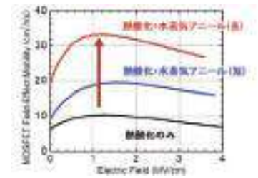
▲ワイドギャップ半導体SiCのMOSFET反転層移動度のアニール処理による向上効果
