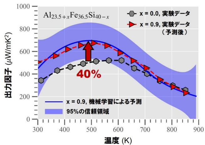
図：(左) 機械学習を取り入れた材料研究開発の流れ、(右) 機械学習を取り入れることにより中温域での出力因子を 40%程度向上させることに成功
