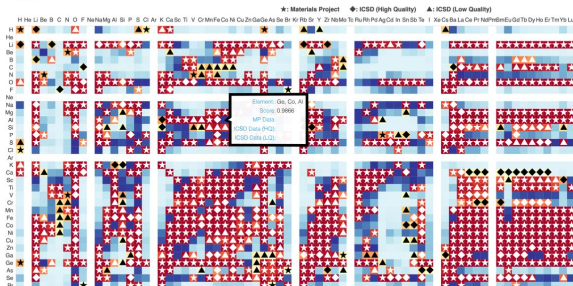
図 1： 元素反応性マップ( https://erm.starrydata.org/ )の一部。Ge,Co,Al の 3 元素のマスをマウスを置いた状態。この例では第 1 元素をゲルマニウム (Ge) としたマップの一部を示しており、横方向が第 2 元素、縦方向が第 3 元素となっています。青色が濃い領域の一つであるコバルト (Co) とアルミニウム (Al) の組み合わせでは、データベースに登録がなかったにもかかわらず、機械学習からは高い反応性スコア 0.9866 が予測され、実験により複数の新物質の合成に成功しました。
