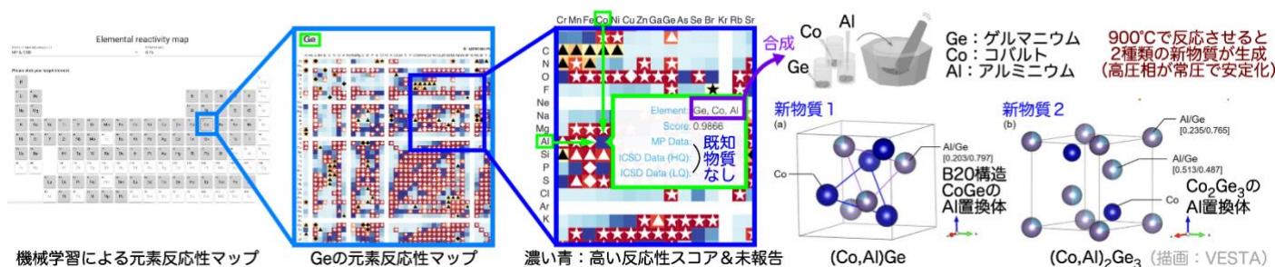
図. 元素反応性マップに基づく新物質探索実験によって発見した2種類の新物質
