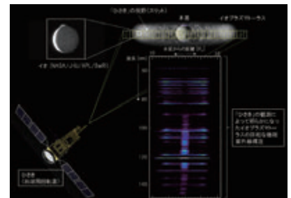
ひさき衛星搭載の極端紫外望遠鏡が捉えた木星近傍のプラズマ発光スペクトル
