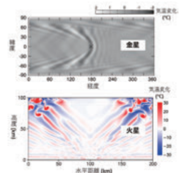
金星の山岳波(上)や火星のダスト嵐で発生する波動(下)など惑星流体力学の数値シミュレーション
