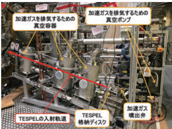
ドイツ・マックスプランク・プラズマ物理研究所のW7-Xに取り付けられたTESPEL入射装置
