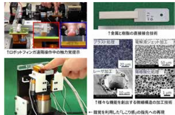
ハプティックデバイスとそれを支える生産加工技術 Haptic devices and manufacturing technologies producing novel devices
