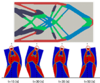
トポロジー最適設計 Topology optimization
