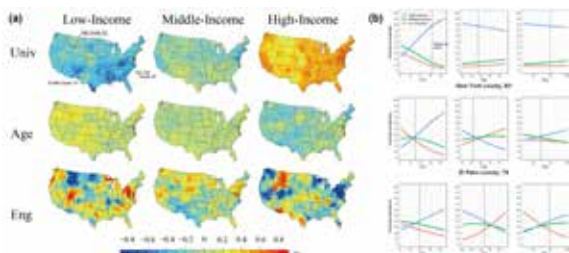
定数と制約と空間的異質性を考慮した空間統計モデルの開発： (a) 準弾力性の空間分布；(b) 予測確率の変化 Spatial statistical models considering constant sum constraints and spatial heterogeneity: (a) spatial distribution of semi-elasticity; (b) changes in predicted probabilities
