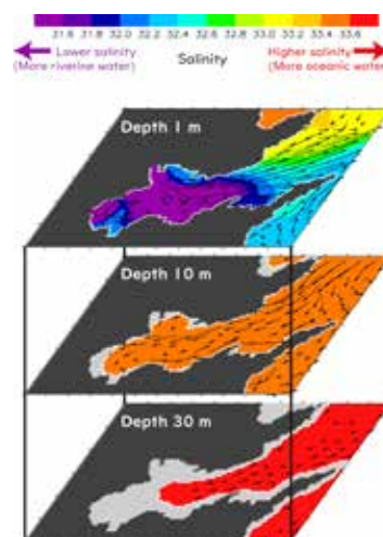
大槌湾の数値モデリング Numerical modeling of Otsuchi Bay
