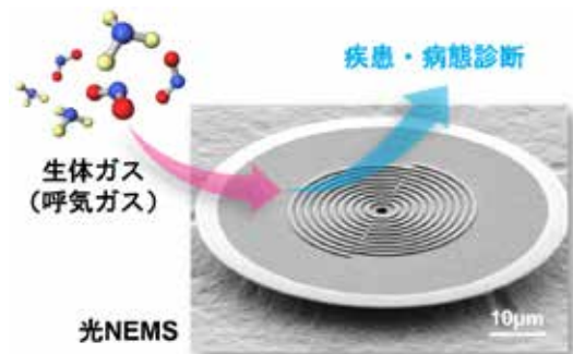
ヘルスケア(呼気診断)用NEMSガスセンサデバイス NEMS gas sensing device for the healthcare (Breath diagnosis)
