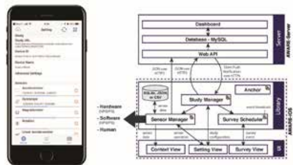
AWARE: コンテキスト認識・モバイルセンシング研究のためのオープンソースのセンシングフレームワーク (フィンランド共和国・オウル大学と共同開発) AWARE: An open-source mobile sensing framework for passive mobile sensing and context recognition research (Collaboration work with the University of Oulu in Finland)
