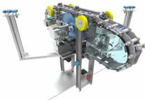
HanGrawler: 無限軌道機構を用いた天井移動ロボット HanGrawler: Large-payload and high-speed ceiling mobile robot using crawler
