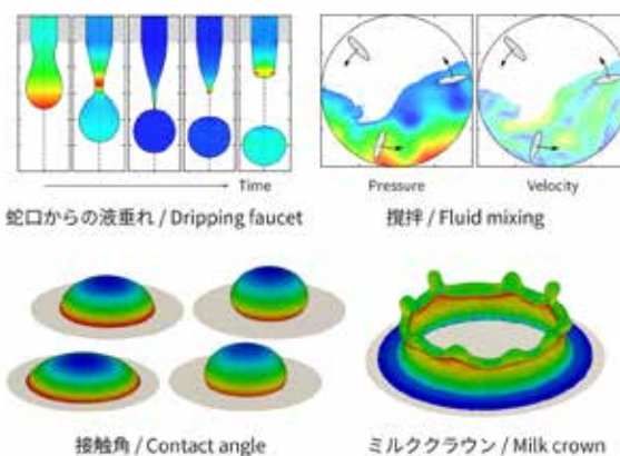
粒子法による流体シミュレーション Fluid simulation using a particle method
